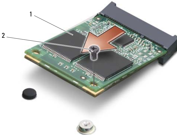
1 scheda FCM 2 vite di fissaggio M2 x 3-mm
