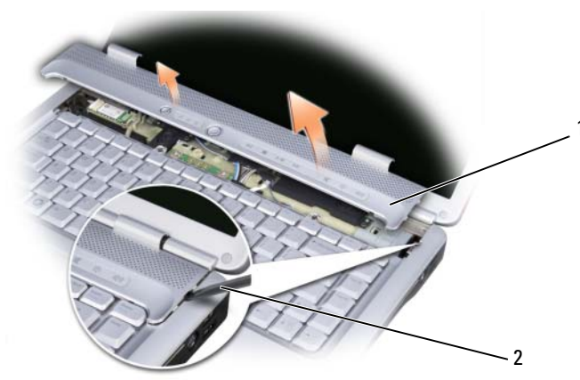
1 coperchio del cardine 2 graffietto
